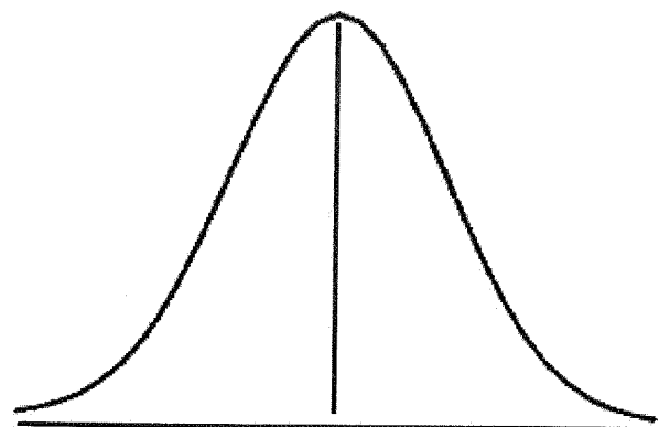
شکل ۱- امکان جمع‌آوری اطلاعات در دو سمت منحنی توزیع نرمال (در غیاب فرضیه)
